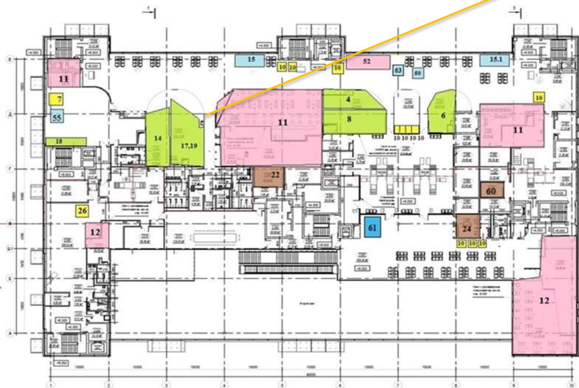
План 2-го этажа (на отм. +6.000). М 1:200
